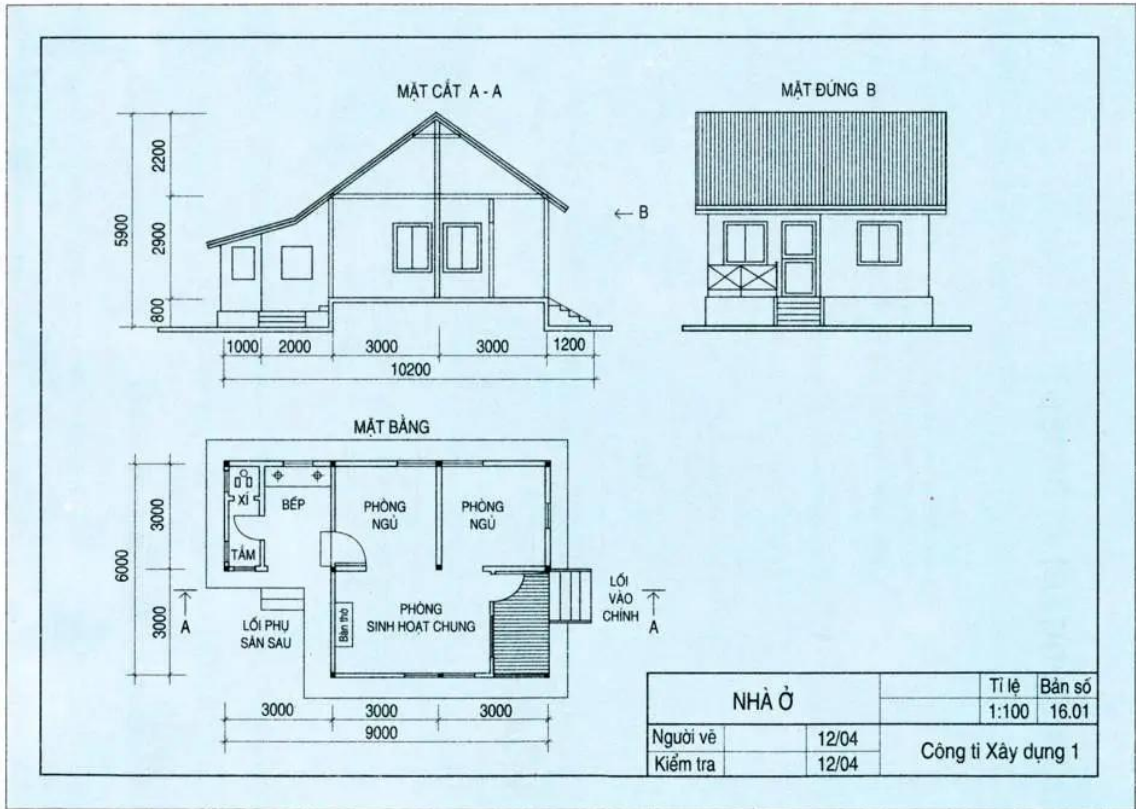
Hình 16.1: Bản vẽ nhà ở
