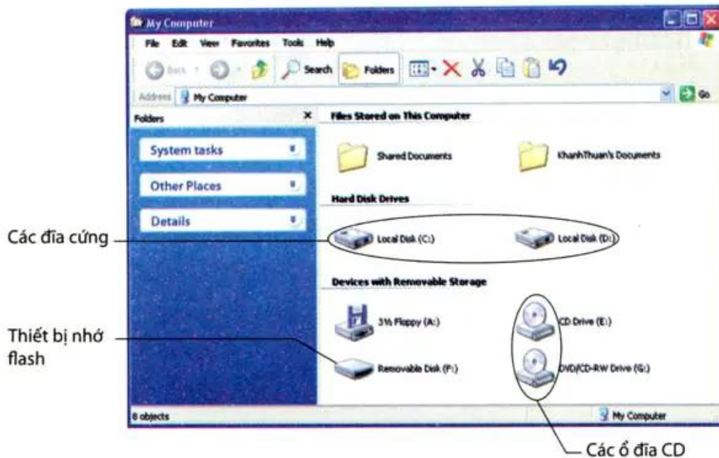
Hình 7. Cửa sổ My Computer
