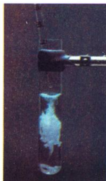
Hình 5.7. Dung dịch AgNO 3 tác dụng với dung dịch NaCl
