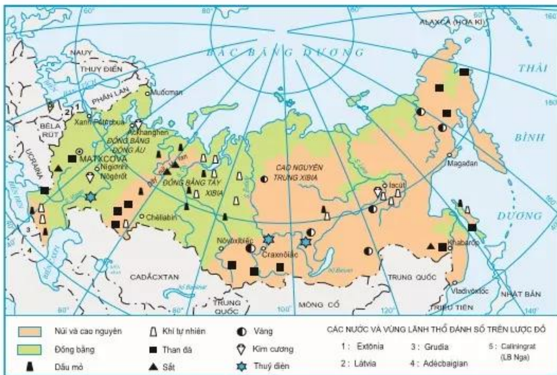
Hình 10.1. Địa hình và khoáng sản LB Nga
